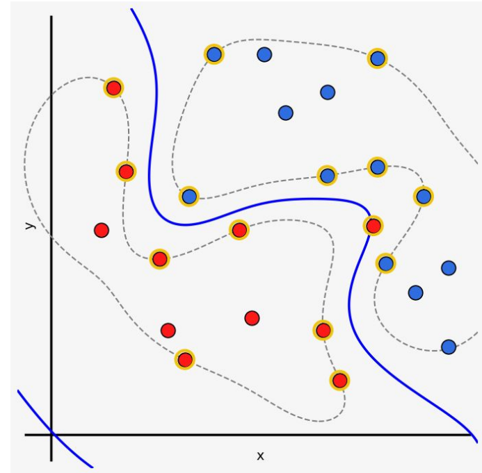
Kernel (RBF)
